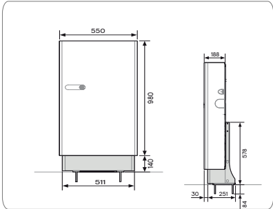
Vloormontage met voetstuk
